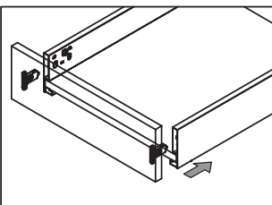
вставить фасад в корпус ящика до щелчка
