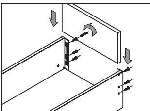
задняя часть
