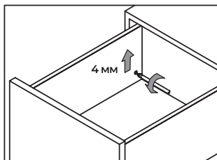
регулировка наклона
