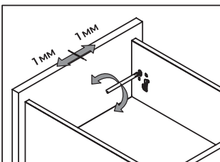
регулировка фасада вправо | влево
