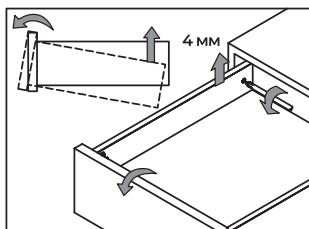
регулировка наклона ящика
